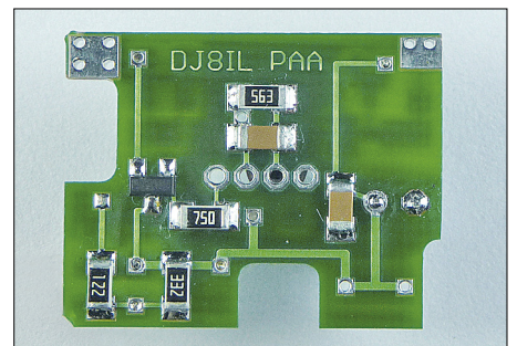
Bild 12: Bestückte Platinenunterseite
