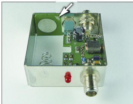
Bild 22: Eingelegte Anschlussplatte für den Pluspol der Lithiumbatterie
