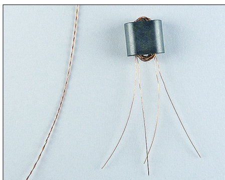
Bild 15: Verdrillter Draht (links) und fertig bewickelter Ringkern (rechts)
