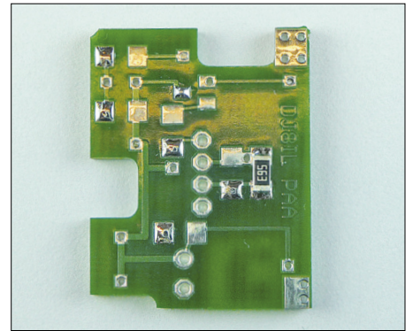
Bild 10: Beispiel für einen vollständig aufgelöteten Widerstand
