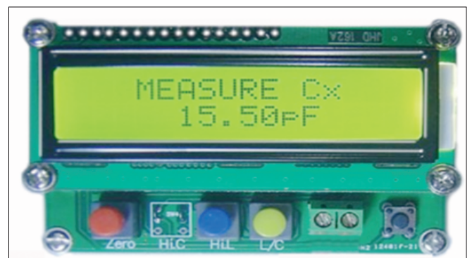
Bild 1: Ansicht des Moduls ohne Anschlussleitungen
